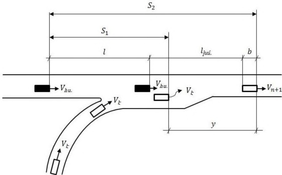
Նկ. 5. Հիմնական ճանապարհի վրա ելքի հաշվարկային սխեման փարանցիկ և միախառնվող ա/մ-ների միջև S_1 հեռավորության որոշման համար:
