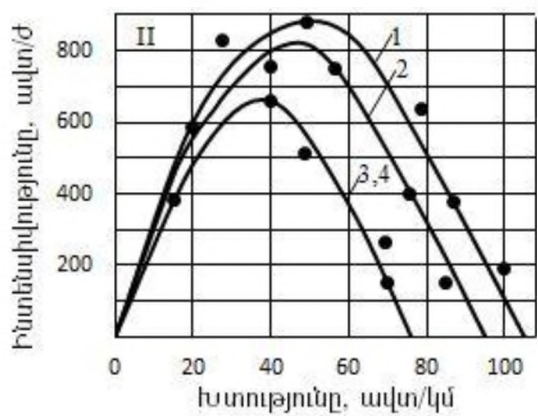
Նկ. 3. Տրանսպորտային հոսքի համար հիմնական կախվածությունները. I' «ինտենսիվություն-արագություն», II' «ինտենսիվություն-խտություն»: ա) մայրուղային փողոցի արտաքին գոյու վրա, բ) «Երեքնուկի փերև» փրանսպորտային հանգույցի ձախ շրջադարձային էջի վրա ( r = 35 մ, i = +35 %):
