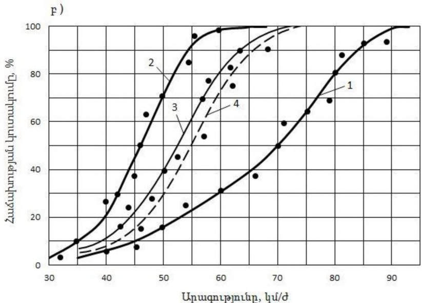
Նկ. 6. Բաշխման (w) և կուտակման (ρ) կորերը որոշ մայրուղային փողոցների համար:
