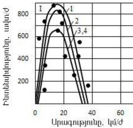
Նկ. 3. Տրանսպորտային հոսքի համար հիմնական կախվածությունները. I' «ինտենսիվություն-արագություն», II' «ինտենսիվություն-խտություն»: ա) մայրուղային փողոցի արտաքին գոյու վրա, բ) «Երեքնուկի փերև» փրանսպորտային հանգույցի ձախ շրջադարձային էջի վրա ( r = 35 մ, i = +35 %):
