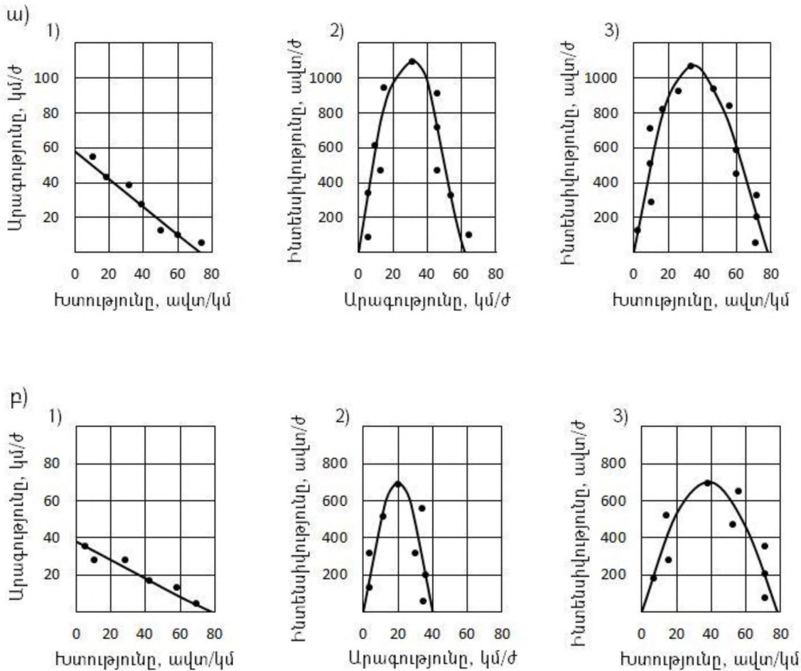
Նկ. 2. Տրանսպորտային հոսքի համար հիմնական կախվածությունները, երբ հոսքում 70 %-ը թեթև մարդափար ավտոմոբիլներ են. ա) ճանապարհի արտաքին գոտու վրա, երբ V_{ազ.} = 60 կմ/ժ և q_{լսճ.} = 72 ավտ/կմ, բ) երեքնուկի տերևի ձախ շրջադարձային էջքի վրա ( R = 60 մ, i = +30\% ), երբ V_{ազ.} = 38 կմ/ժ և q_{լսճ.} = 79 ավտ/կմ: 1-«արագություն-խտություն» կախվածություն, 2-«ինտենսիվություն-արագություն» կախվածություն, 3-«ինտենսիվություն-խտություն» կախվածություն:
