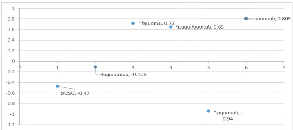
Գծապատկեր 1. Պիրսոնի կոռելյացիայի գործակից
