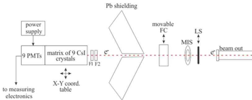
Рис. 13. Схема эксперимента в зоне калибровки кристаллов. MIS – магнитоиндукционный датчик; LS – люминофорный экран; F1, F2 – пластиковые сцинтилляционные счетчики пальчикового типа.
