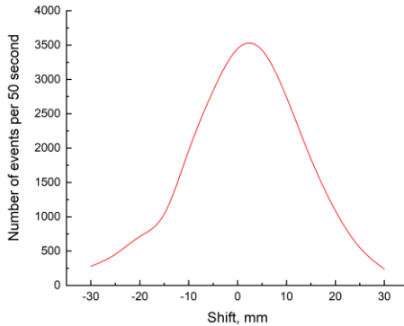
Рис. 12. Горизонтальный профиль пучка экстремально низкой интенсивности со средней энергией 40 МэВ на выходе тракта в зоне тестирования кристаллов.
