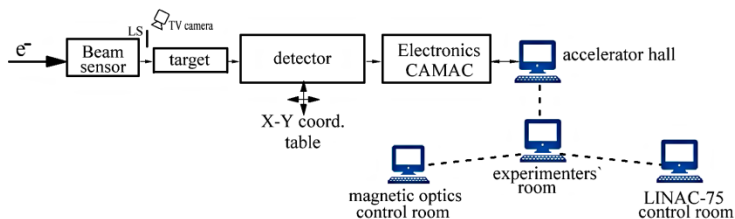
Рис. 15. Типовая блок-схема измерительной аппаратуры, используемой на линейном ускорительном комплексе ЛУЭ-75; LS – дистанционно-перемещаемый люминофорный экран, используемый при настройке магнитной оптики.
