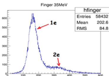
Рис. 14. Гистограмма распределения числа событий по каналам АЦП при энергии электронов 35 МэВ.
