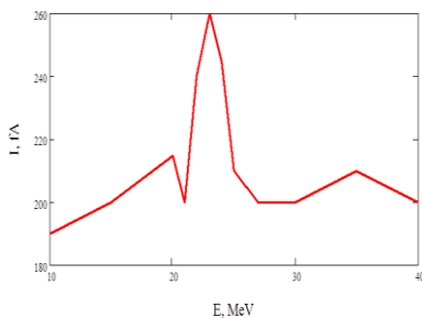
Рис. 10. Спектр темнового тока при работе только 1-го клистрона.
