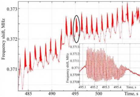
Նկ. 2.4: Քնային զարկերակի սֆիզմոգրամը, որը գրանցված է միաշերտ հարթ կոճի վրա հիմնված մեխանիկական տատանողական համակարգով վիբրացիոն տվիչով: Սֆիզմոգրամի վրա վերադրված է պարբերականորեն կրկնվող ձայնարկման արդյունքում առաջացող բարձրհաճախային բաղադրիչը: Ներդիրը ցույց է տալիս ձայնարկման ակտիվության ընդլայնված մեկ հատված:
