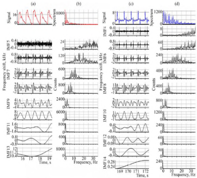
Նկ. 2.6: Քնային զարկերակից վիբրացիոն (a, b) և ակուստիկ (c, d) միաշերտ հարթ կոճերի վրա հիմնված տվիչներով գրանցված սֆիգմոգրամները և դրանց հզորության սպեկտրները, սեփական ներքին մոդային ֆունկցիաները (a, c), և դրանց սպեկտրները՝ ազդանշանները էմպիրիկ մոդային տրոհման ենթարկելուց հետո:
