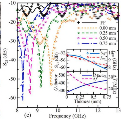
Նկ. 12: Ընդհատված Գուբաուի գծի (ԳԳ) հետ ինտեգրացված վեկտորային ցանցային անալիզատորի թեստավորման կառուցվածքի և հետազոտվող ձողի (a) լուսանկարը և (b) սխեման: (c) Միկրոալիքային անցման S_{21} գործակցի արժեքները պղնձե ձողի համար (1.5մմ տրամագծով և 25մմ երկարությամբ) շրջապատող դիէլեկտրիկ շերտի տարբեր հաստություններով: Սև գիծը ներկայացնում է համակարգն առանց պղնձե ձողի, այսինքն միայն ընդհատված ԳԳ-ն: Վերին ներդիրը ցույց է տալիս S_{21} նվազագույնի և ռեզոնանսային հաճախության կախվածությունը դիէլեկտրիկ շերտի հաստությունից: Մոդելավորման տվյալները պատկերված են կետային նշանների միջոցով, իսկ փորձարարական տվյալները նշված են գծերով: Ստորին ներդիրը ցույց է տալիս համակարգի բարորակության և թողունակության կախվածությունը դիէլեկտրիկ շերտի հաստությունից:
