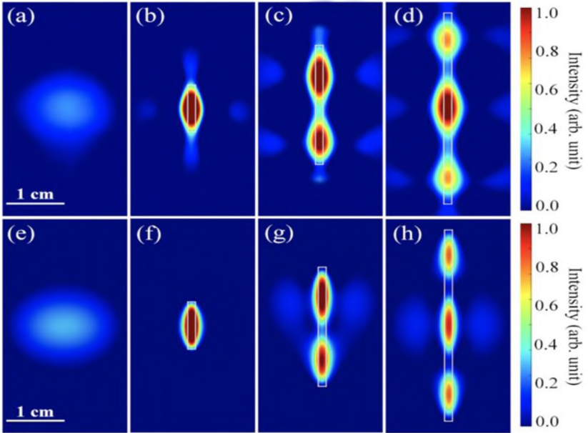
Նկ. 10: Ընկած գծային բևեռացված միկրոալիքային էլեկտրամագնիսական դաշտի բաշխվածությունը 10 ԳՀց հաճախությամբ (a) գրանցված և (e) մոդելավորված: (b)–(d) գրանցված և (f)–(h) մոդելավորված ՄՄՄԴ-ի բաշխվածությունները պղնձե ձողի շուրջ 1,5 մմ տրամագծով և համապատասխան երկարություններով (b), (f) 10 մմ, (c), (g) 25: մմ, (d), (h) 40 մմ նմուշից 1 մմ հեռավորության վրա: Մոխրագույն ուղղանկյունները նկարագրում են պղնձե ձողերի եզրերը:
