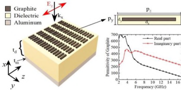
Նկ. 1: Պարբերական կառուցվածքի 3D տեսք, որը բաղկացած է այլումինե շերտից, դիելեկտրիկ շերտից և ուղղանկյուն գրաֆիտի ժապավեններից կազմված պարբերական կառուցվածքից, գրաֆիտի դիելեկտրիկ թափանցելիության իրական ( \epsilon' ) ու կեղծ ( \epsilon'' ) մասերը կախված հաճախությունից
