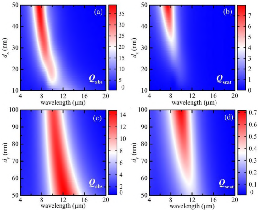
Նկ. 6: Կլանման (առաջին սյունակ) և ցրման (երկրորդ սյունակ) արդյունավետությունները՝ որպես ֆունկցիա ալիքի երկարությունից և (a-b) d_x և (c-d) d_y չափերից:
