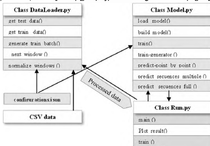
Գծապատկեր 2. Գործարկման դաս-մոդելի գծապատկերը
