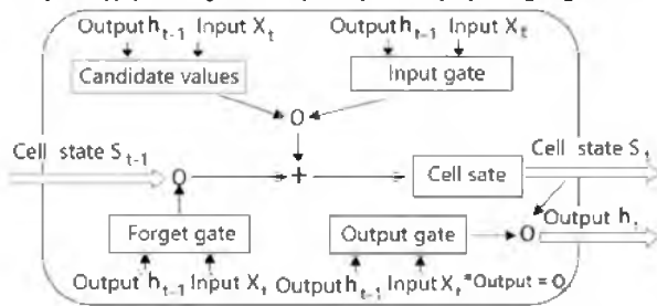
Գծապատկեր 1. LSTM հիշողության բջջի ընդհանուր կառուցվածքը
