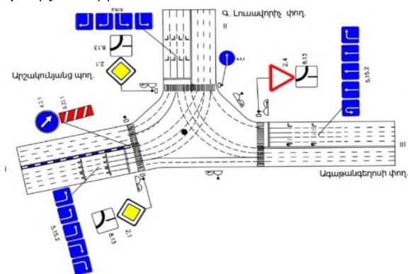
Նկ. 1 Արշակունյաց պ. – Ագաթանգեղոս փ. – Լուսավորիչ փ. խաչմերուկի երթևեկության կազմակերպման սխեման
