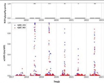
Նկար 2. Բոլոր 700 պատկերների դիֆարկում՝ Սևանա լճի RGB վրա հիմնված ծաղկման հայտնաբերման համար (վերև) և ՎՋԾ հիմնված դասակարգում (ներքև)
