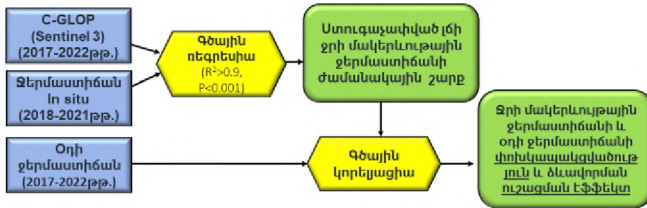
Նկար 2. ՋՄՋ ԱՀ և օդի ջերմաստիճանի հեղ փոխազդեցության միջդարեկան և ներդարեկան առանձնահատկությունների վերլուծության համառոտ սխեման
