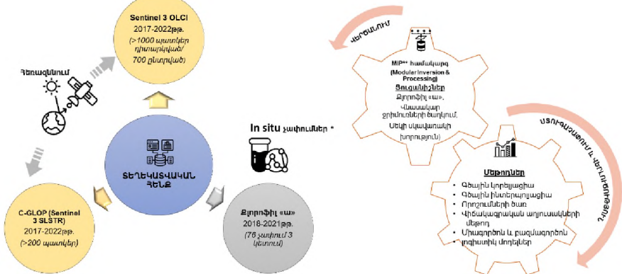
Նկար 4. Լճի ծաղկման մեթոդական մոդեցման մշակման տեղեկատվական հենքը
