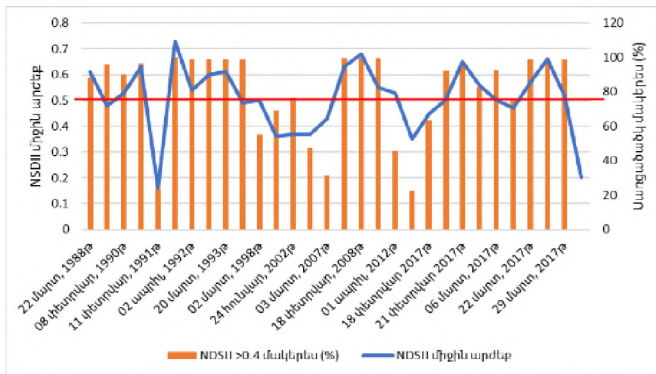
Նկար 1. Սևանա լճի սառցածածկի NDSII արժեքները և լճի սառցապատ մակերեսը՝ ըստ Landsat և Sentinel 2 արբանյակային պատկերների
