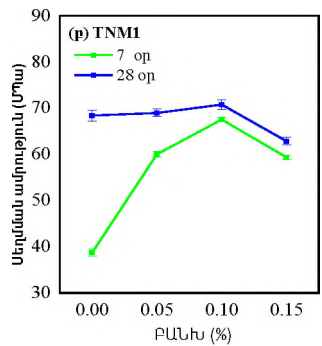
Նկար 3. ա) TNM0, բ) TNM1 և գ) TNM5 ԲԱՆԻ -ներով փորձանմուշների սեղմման ամրությունները 7 և 28 օրական ամրացման հասակում
