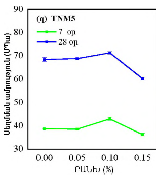
Նկար 3. ա) TNM0, բ) TNM1 և գ) TNM5 ԲԱՆԻ -ներով փորձանմուշների սեղմման ամրությունները 7 և 28 օրական ամրացման հասակում
