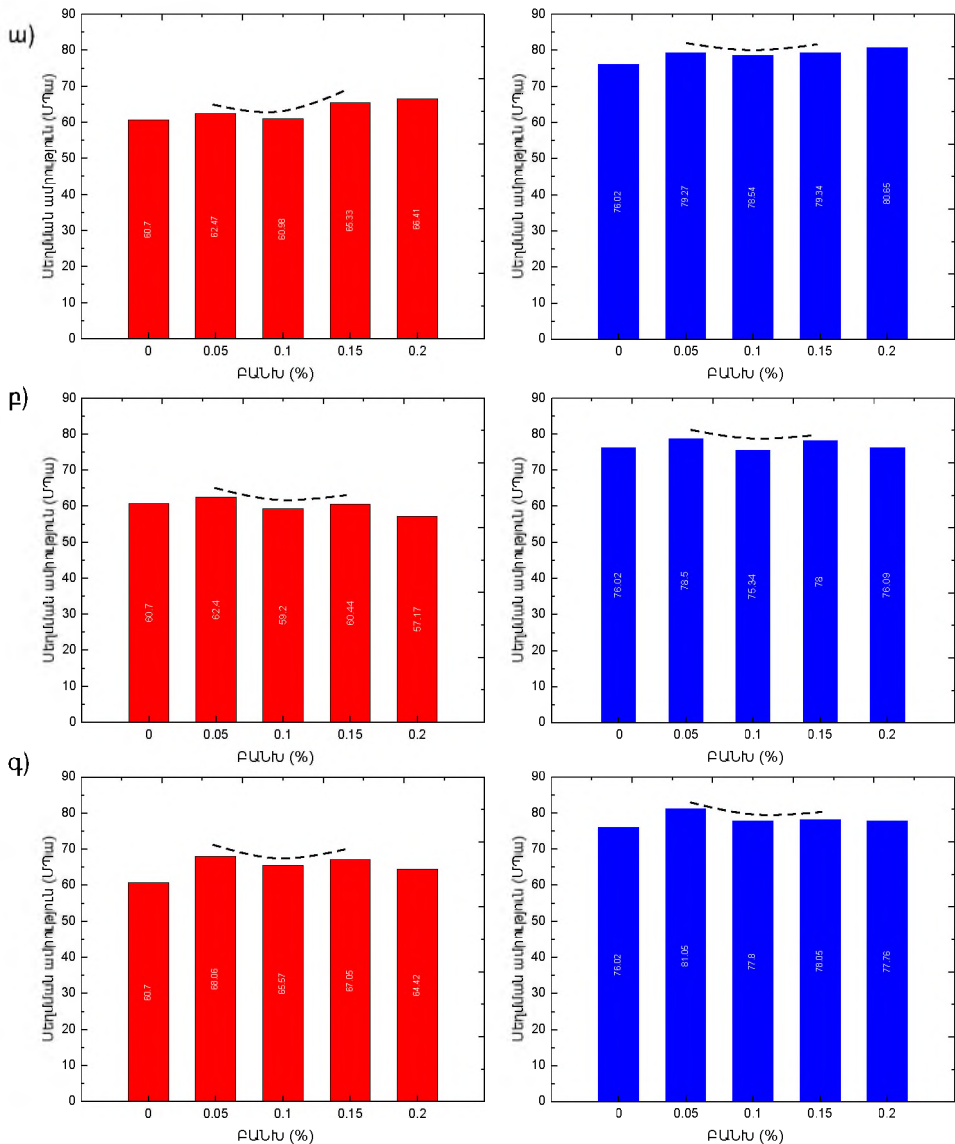
Նկար 6. ա) TNM2, բ) TNM3 և գ) TNM7 տեսակի ԲԱՆՆ -ներով նմուշների սեղմման ամրությունները (7 և 28 օրական)
