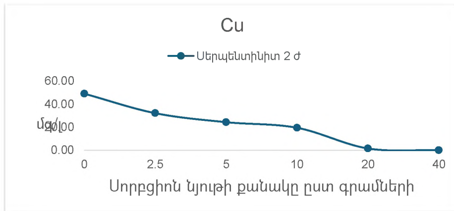
Նկ. 5 Պղնձի կորզումը կախված կիրառվող սերպենտինի քանակությունից 5 ժամվա ընթացքում:
