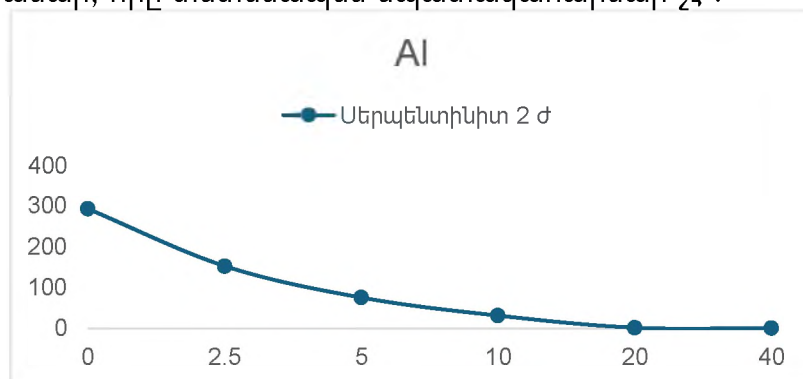
Նկ. 4 Ալյումինի կորզման կախվածությունը կիրառվող սերպենտինիտի քանակությունից 5 ժամվա ընթացքում:
