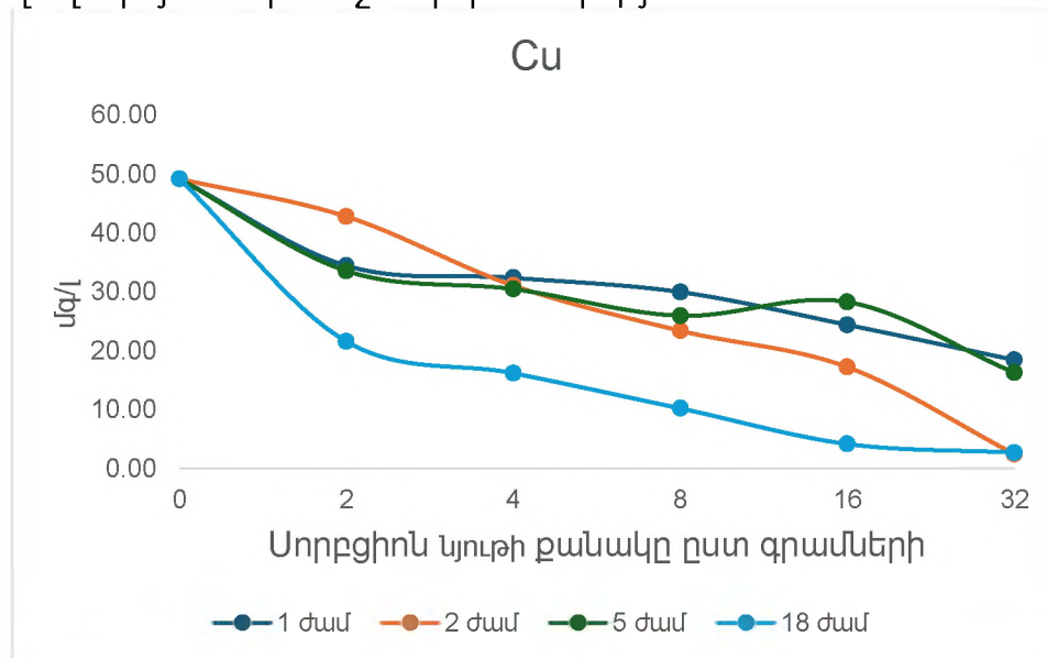
Նկ. 2 Պղնձի կորզումը կախված կիրառվող շլամի քանակությունից. 1 , 2, 5 և 18 ժամ ազդեցության դեպքում
