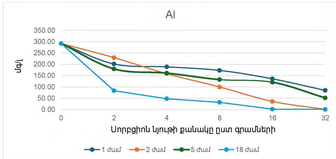
Նկ. 1 Ալյումինի կորզումը կախված կիրառվող շլամի քանակությունից. 1 , 2, 5 և 18 ժամ ազդեցության դեպքում
