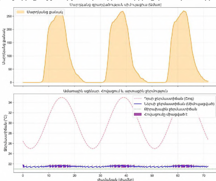
Նկ.2. Ամառային շրջանի կլիմայավորման համակարգի աշխատանքային ռեժիմի սիմուլյացիա՝ օգտագործողների զբաղվածության, արտաքին և ներքին ջերմաստիճանների դինամիկա
