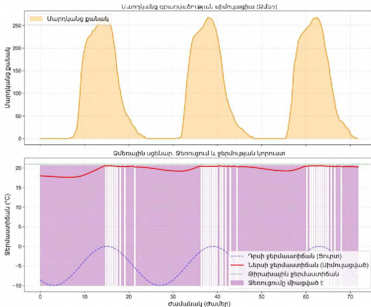
Նկ.1. Ձմեռային շրջանի ջեռուցման համակարգի աշխատանքային ռեժիմի սիմուլյացիա՝ օգտագործողների զբաղվածության, արտաքին և ներքին ջերմաստիճանների դինամիկա
