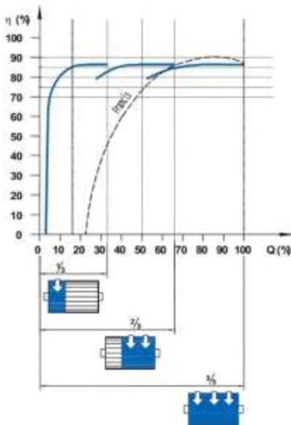
Նկ. 2 Երկսեկցիոն հոսքային տուրբինի օ.գ.գ. կորը
