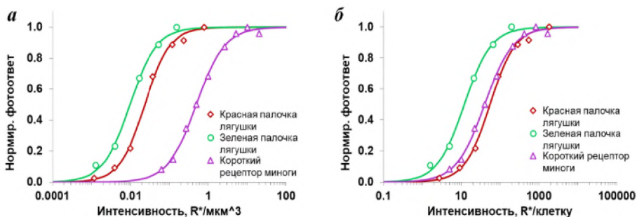
Рис. 2. Оценка абсолютной чувствительности различных фоторецепторов при пересчете интенсивностей светового стимула в число фотоизомеризаций молекул зрительного пигмента на единицу объема (а), и на целую клетку (б). Точки – данные по репрезентативным клеткам, сплошные линии – аппроксимация с помощью функций Хилла.
